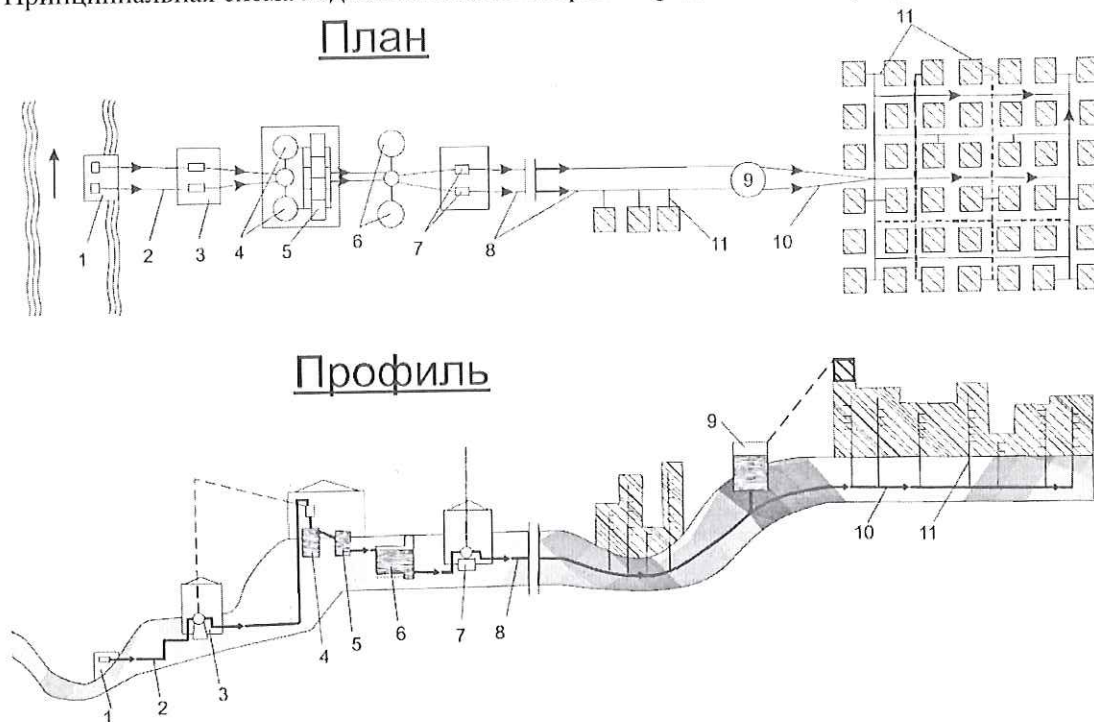
Рисунок 2. Принципиальная схема водоснабжения г. Мирный
