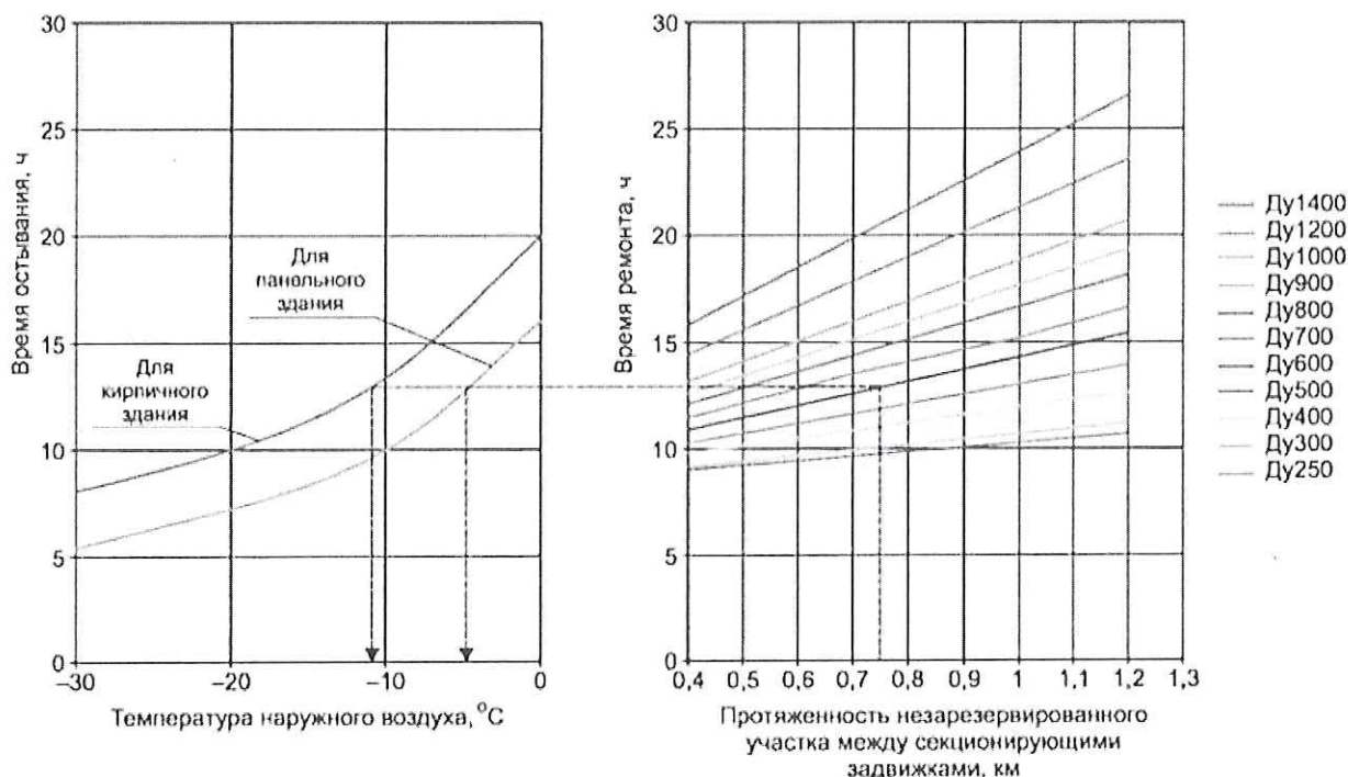
Рисунок 4. Номограмма для определения периодов остывания угловых жилых помещений кирпичных и панельных зданий со снижением температуры внутреннего воздуха помещений с +20 до +12 °С
