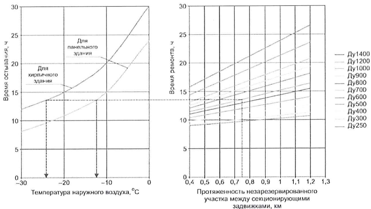
Рисунок 5. Номограмма для определения периодов остывания для подъездов и лестничных клеток жилых зданий со снижением температуры с +15 до +3 °C
