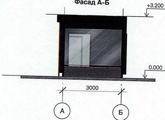
Фасад А-Б
