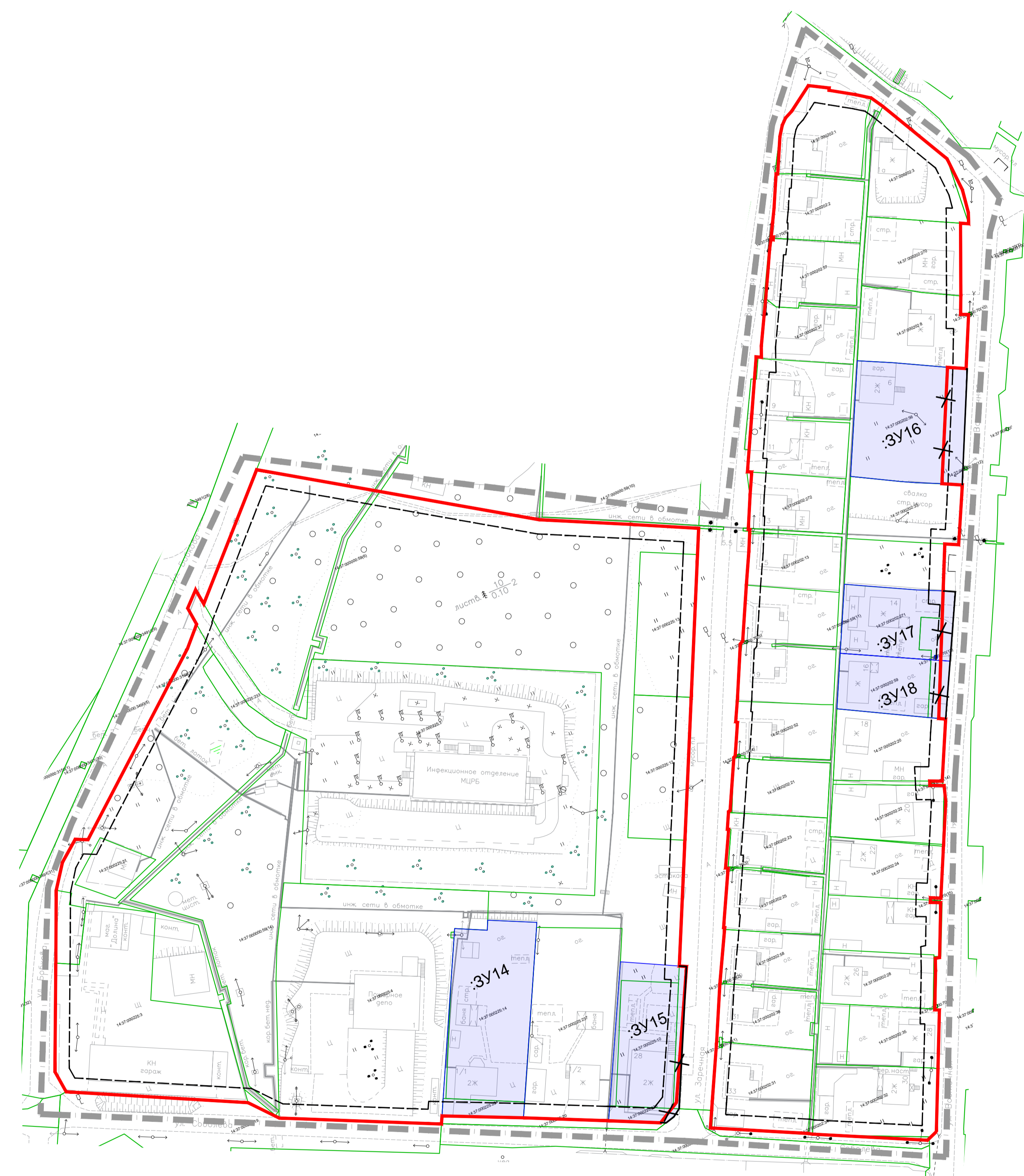
Чертеж межевания территории 2 этап
